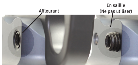
Fig. 10 Installation appropriée de la vis de pression
