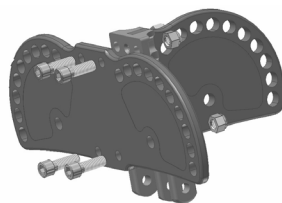
Fig. 20 Fixation de la demi-plaque à la plaque principale
