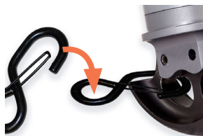
Fig. 14 : Crochet d'entrave se connectant à l'œil d'un autre crochet
